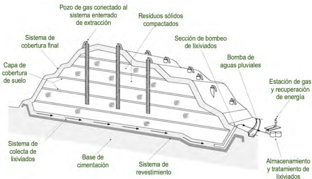
Figura 4. Descripción general de los principales componentes de los rellenos sanitarios (Modificado de Townsend et al., 2015).
