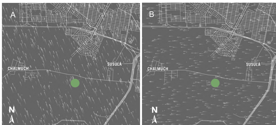
Figura 16. Captura de animación de partículas del día 18 de junio de 2024 a las (A) 20:57 y (B) 11:22 h, indicando la dirección del viento típica de la región: ESE (este-sureste) y E (este) en la zona de estudio. Imágenes tomadas de la aplicación Apple Inc. (2024). Clima (Versión 5.1.0) [Aplicación móvil]. Apple.
