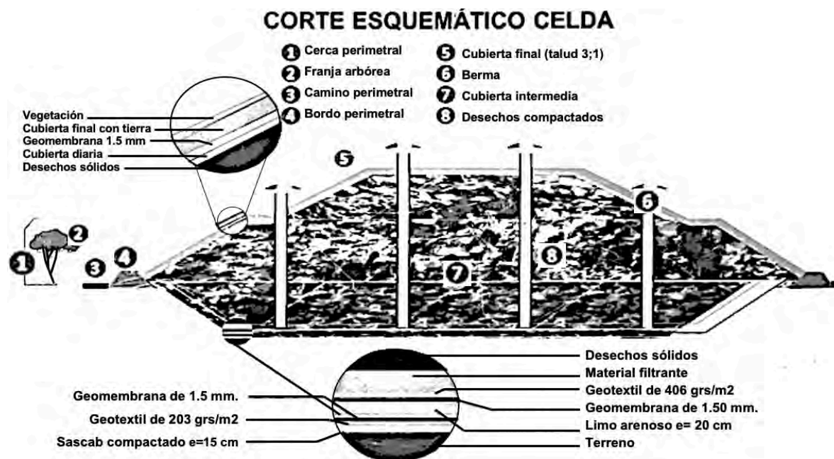
Figura 5. Diagrama de la estructura del relleno sanitario de Mérida (Veolia, 2024).
